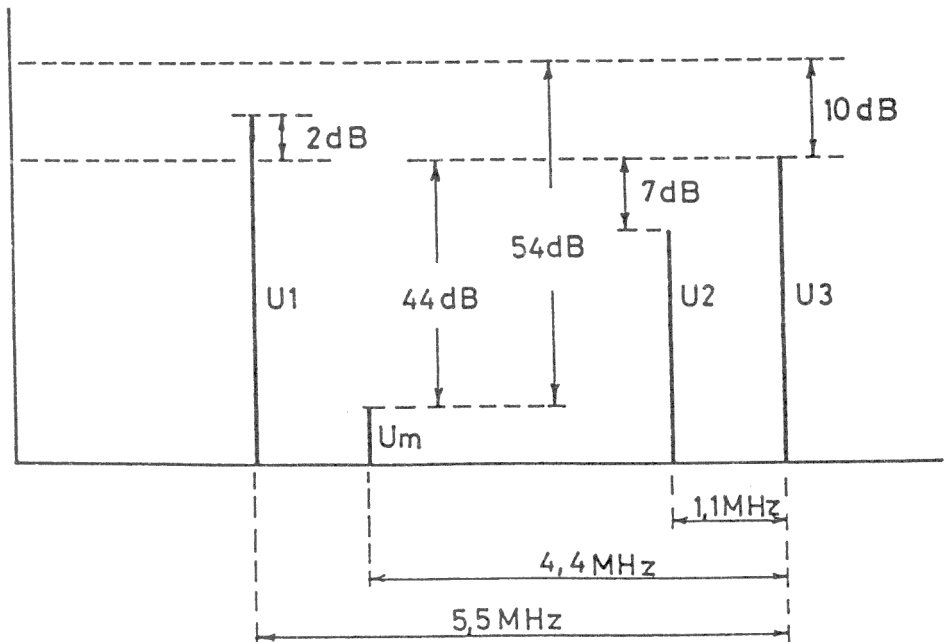
Mynd 2. Tíðniróf á útgangi magnarans.
