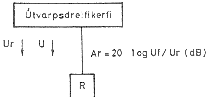
Mynd 2. Endurkastsdeyfung í kerfi.
