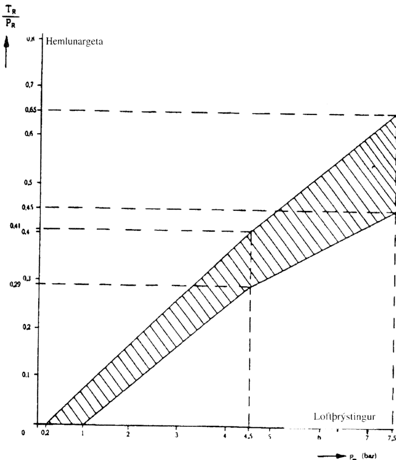
Mynd 6.3: Línurit fyrir festivagn.
